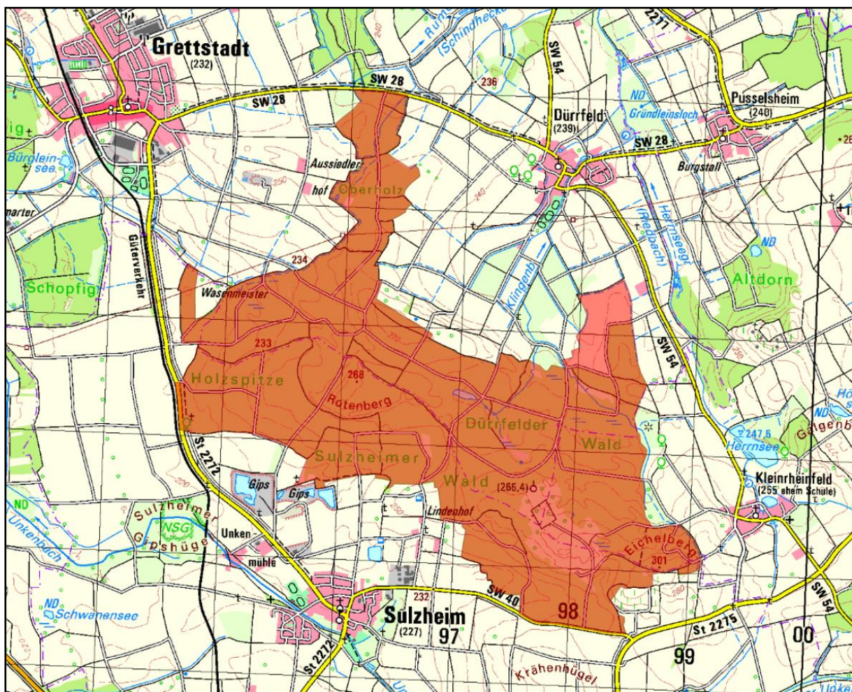
Abb. 1: Übersichtskarte des FFH-Gebiets 6028-371 Dürrfelder und Sulzheimer Wald (ohne Maßstab, Geobasisdaten: BAYERISCHE LANDESVERMESSUNGSVERWALTUNG)
